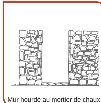
Mur hourdé au mortier de chaux
